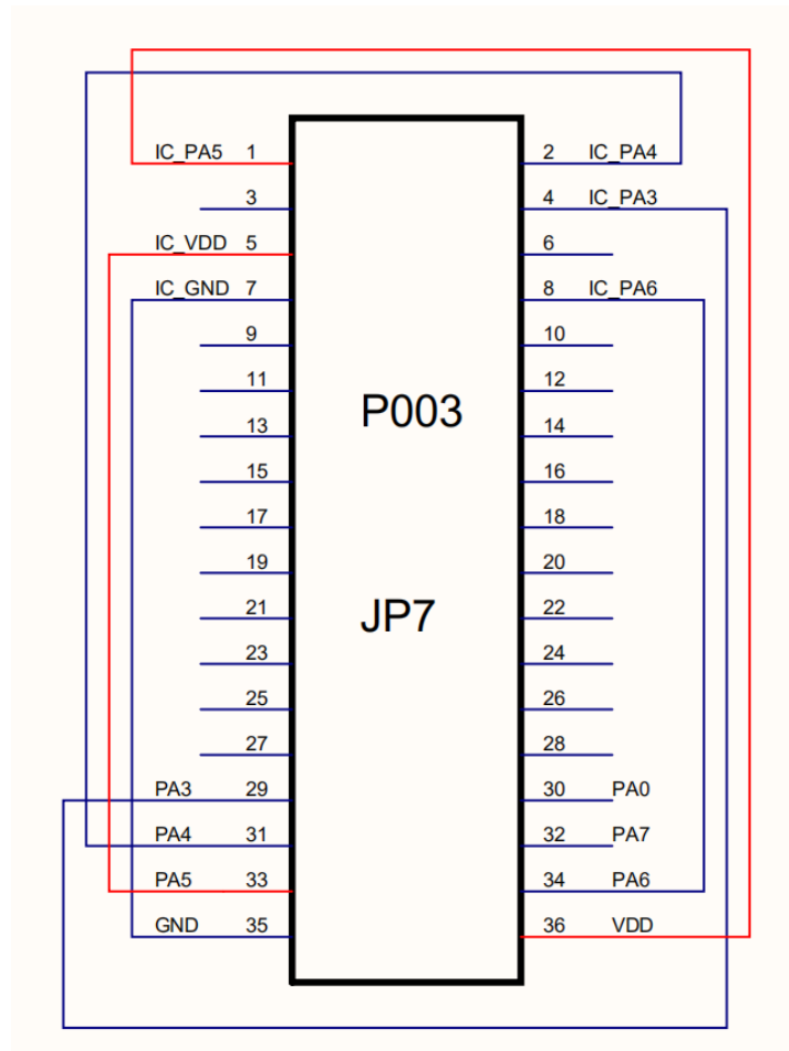
图 21: 使用 P003 时, PMS161-S08B JP7 跳线原理图
